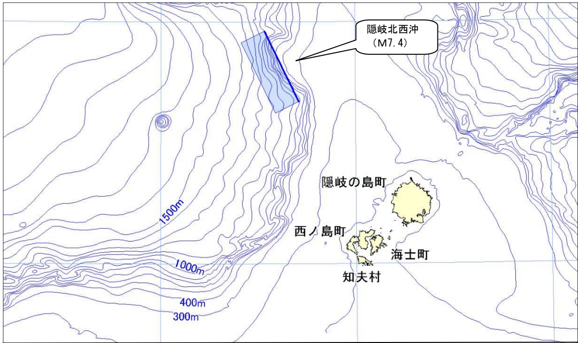
地震動想定対象地震 位置図 その1
