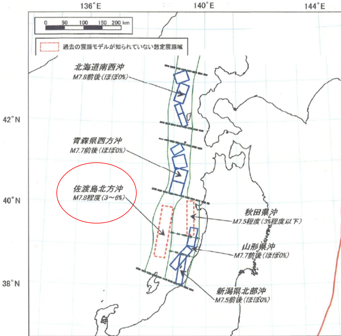
想定地震の震源域・規模および30年確率
