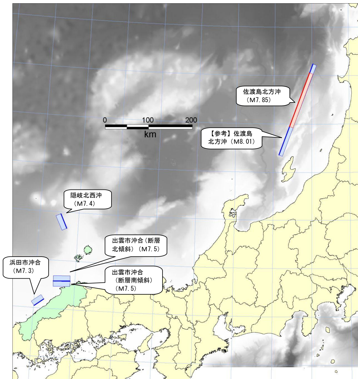
津波の計算を行った想定断層の位置
