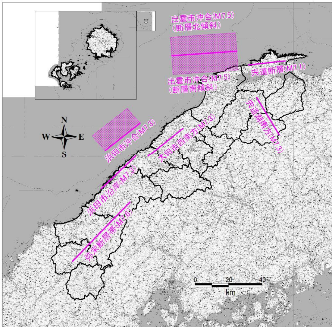
地震動想定対象地震 位置図 その2
