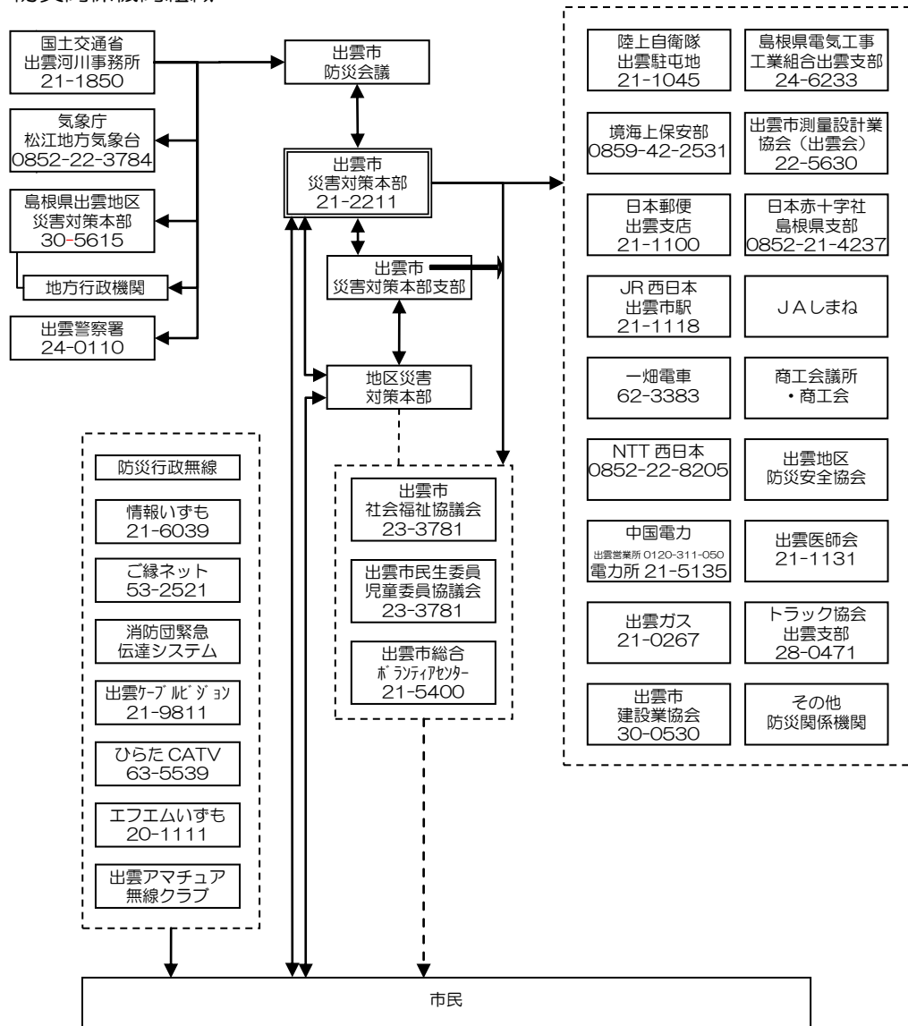
第1図 防災関係機関組織
