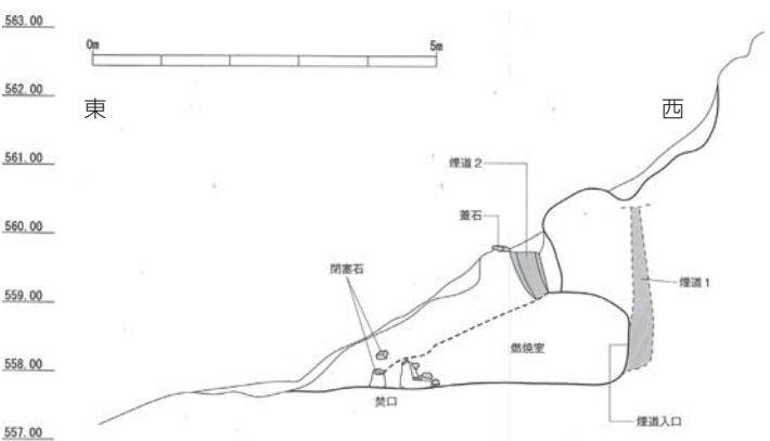
遺構断面見通し図
