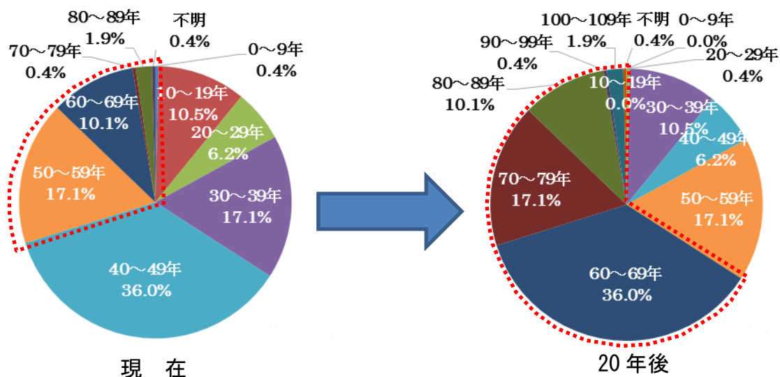
図2 美郷町が管理する道路橋の経過年数ごとの橋梁数
