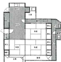
1階平面図
