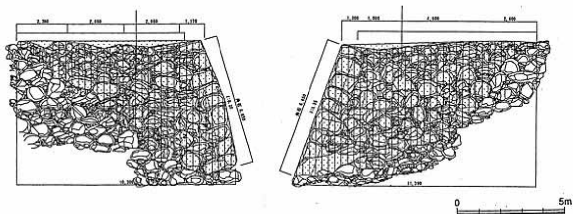
図6 松江城 A本丸北東角石垣 松江市教委2007から
