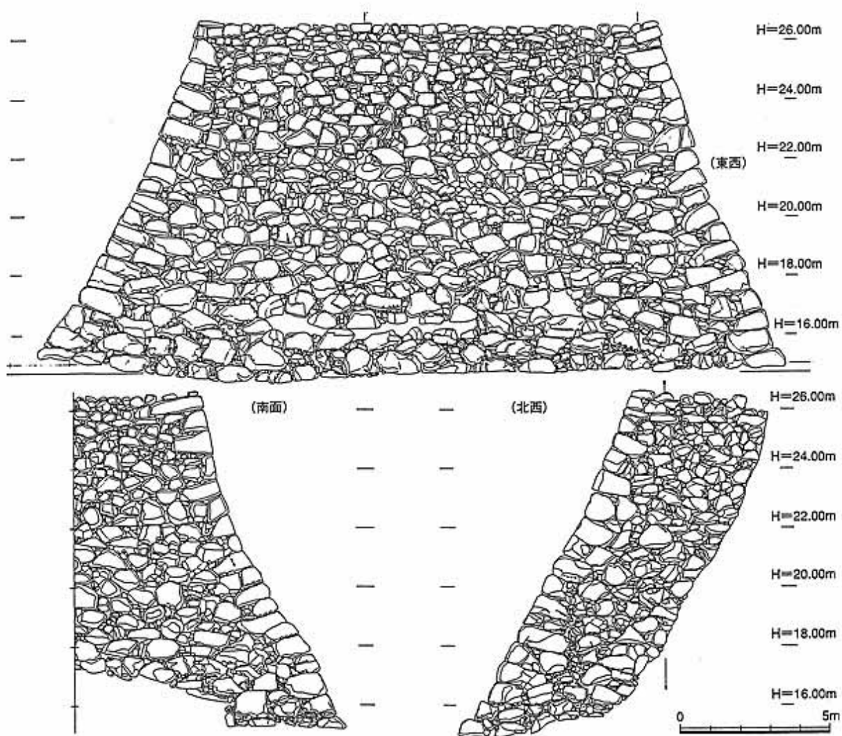
図5 松江城 K-L本丸南東武具櫓の石垣 松江市教委2007から
