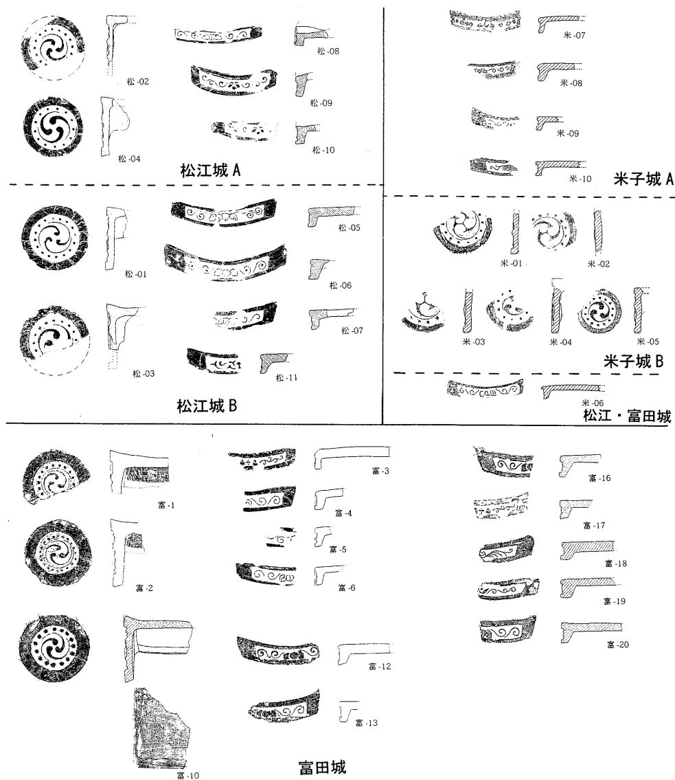
図7 胎土分析した瓦の実測図
