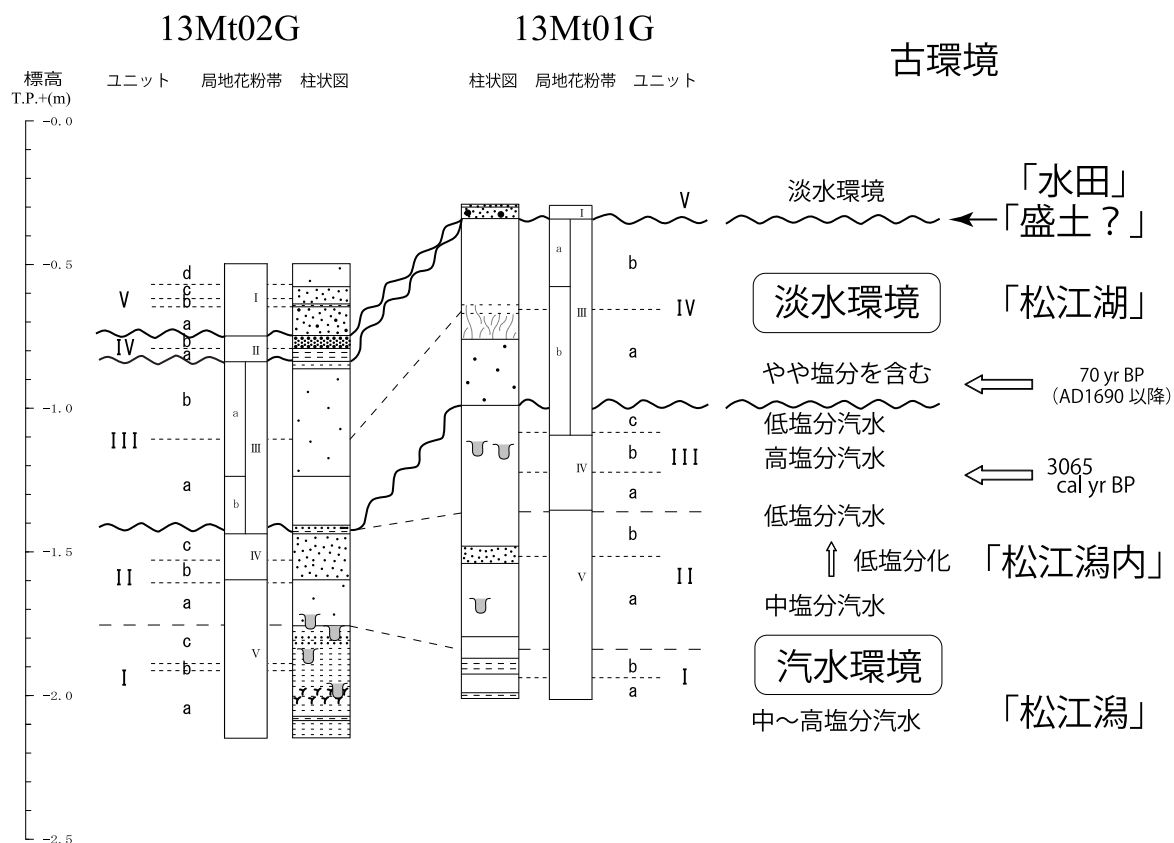
図4 13Mt01Gコアと13Mt02Gコアの対比と古環境 (瀬戸ほか(2015)に、加筆・修正)
