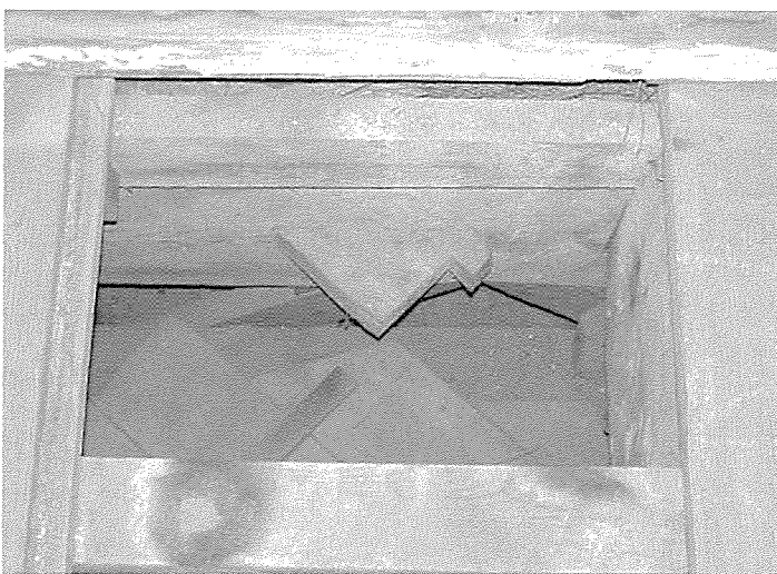
▲写真8 解体状況（解体箇所③）火打材の柄の状況.
