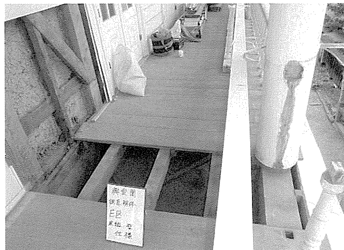
▲写真6 解体状況（解体箇所②）北側中央部壁面をみる。
