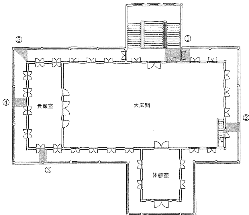
2 階平面図（解体箇所位置図）
