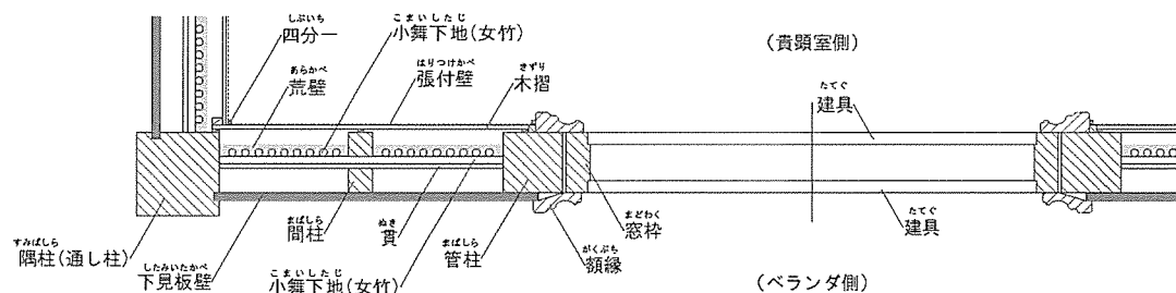
▲B. 貴頭室入側周り断面図
