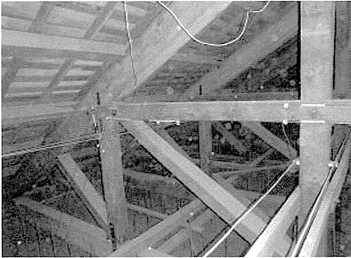
▲真束周辺をみる
