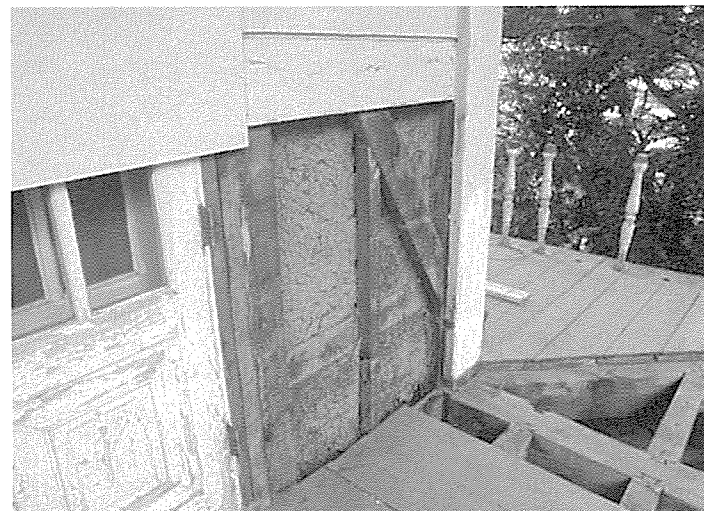
▲写真12 解体状況（解体箇所⑤）ベランダ南西隅壁面
