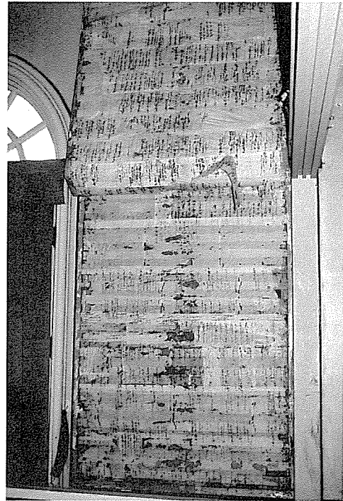
写真2 壁紙をめくった様子
