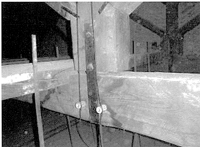
▲陸梁と真束の箱金物
