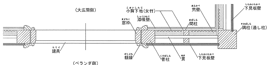
▲A. 入側周り壁断面図
