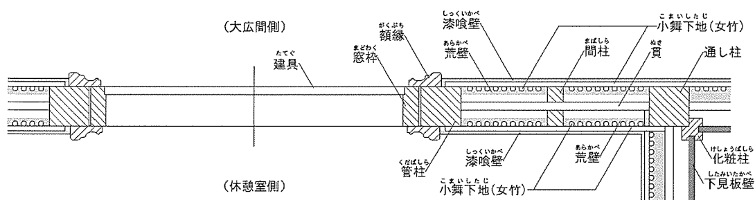
▲C. 間仕切壁断面図
