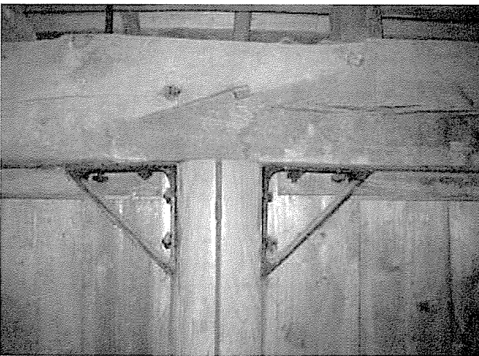
▲側柱（円柱）と敷桁
