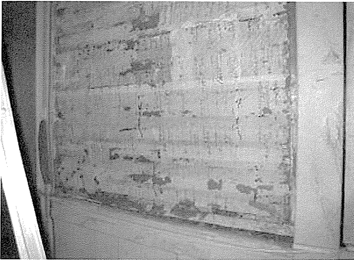
▲貴顕室張付壁下地
