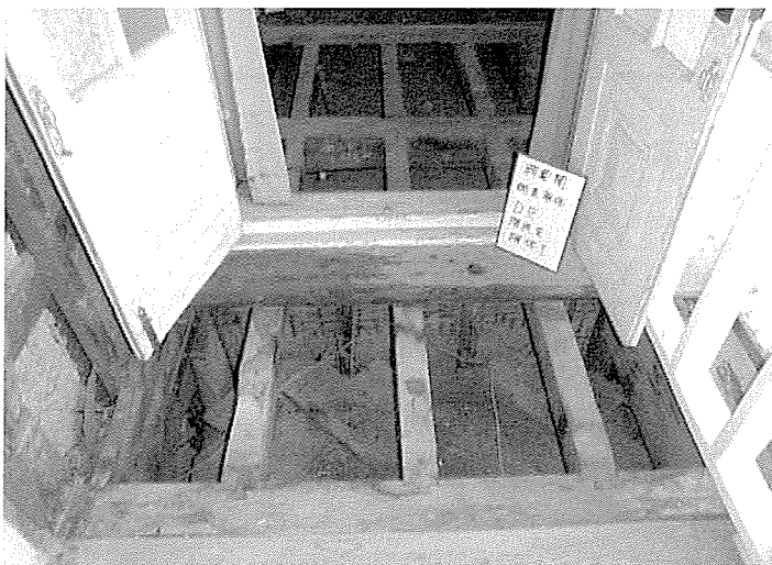
▲写真3 解体状況（解体箇所①）階段室北側のペランダを見る。
