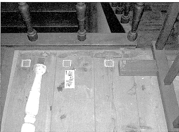
▲写真2 解体状況（解体箇所①）床板の痕跡を見る。
