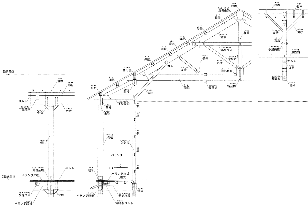
▲小屋組構造図
