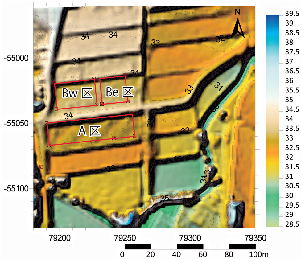
図2 SLAM測量より作成した測量図と 地中レーダ探査範囲
