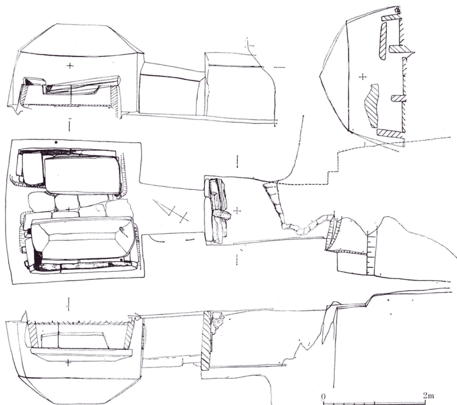
第6図 北小原横穴実測図
