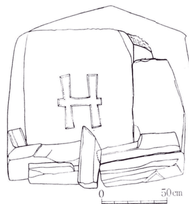
第7図 閉塞石正面図
