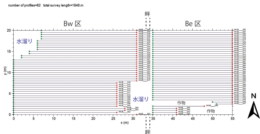
図 4 B 区における測線配置図
