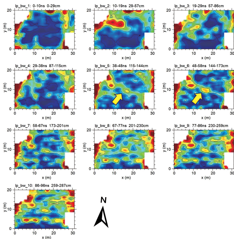
図6 Bw区におけるtime-slice図
