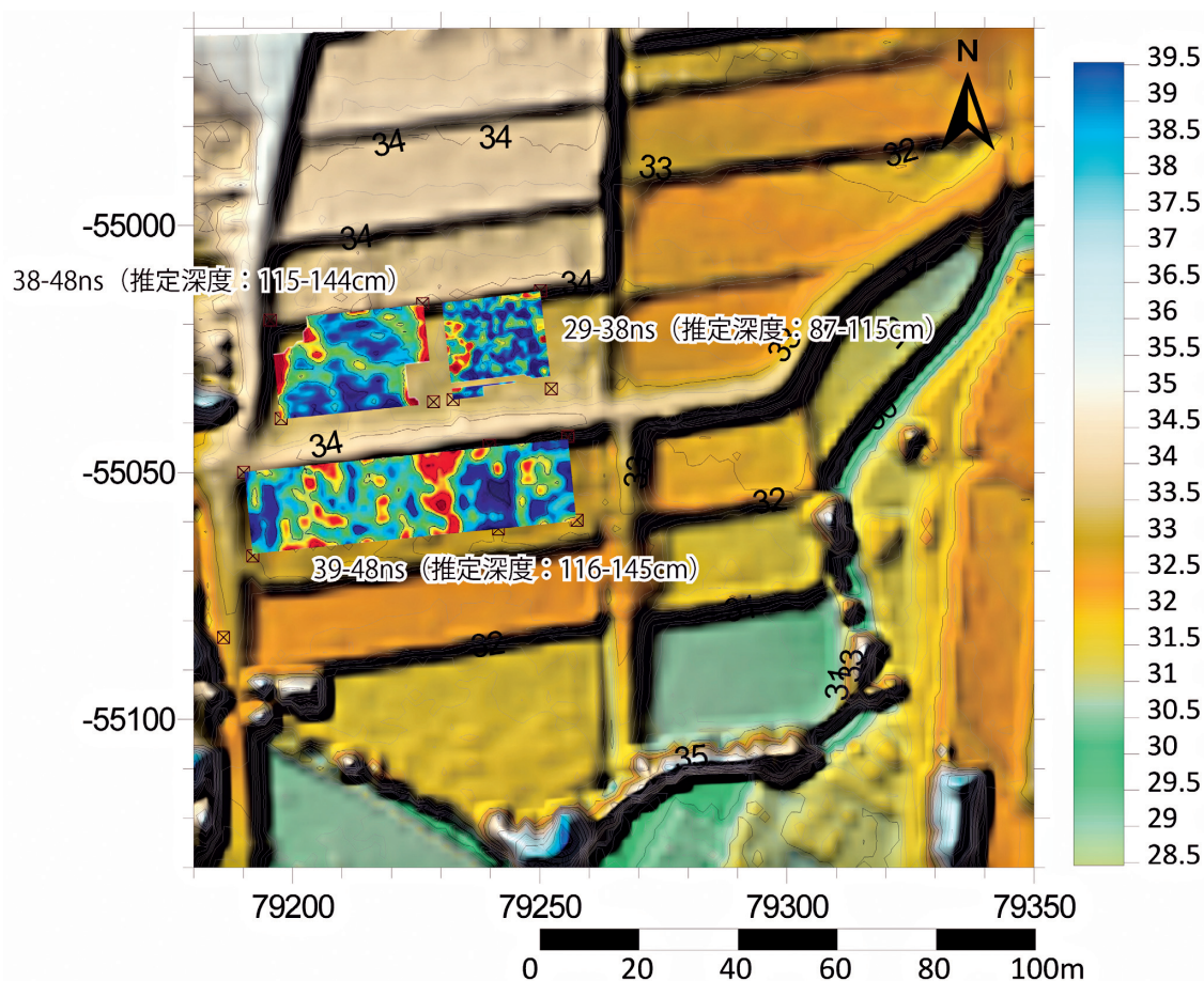
図8 平ノ前廃寺における代表的な地中レーダ探査結果
