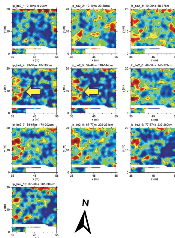
図7 Be区におけるtime-slice図
