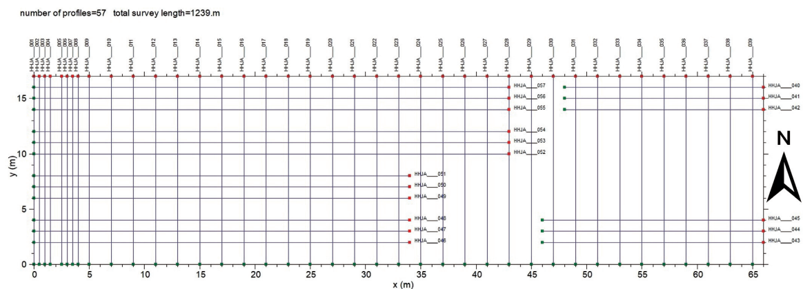
図 3 A 区における測線配置図
