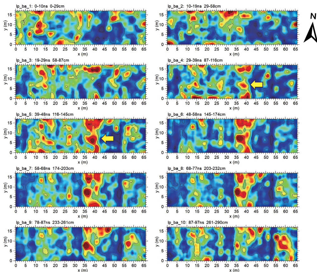
図5 A区におけるtime-slice図
