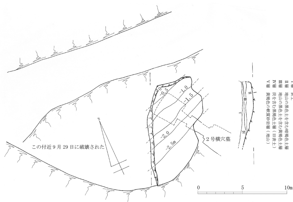
図10 2号横穴墓と後背墳丘の位置関係図
