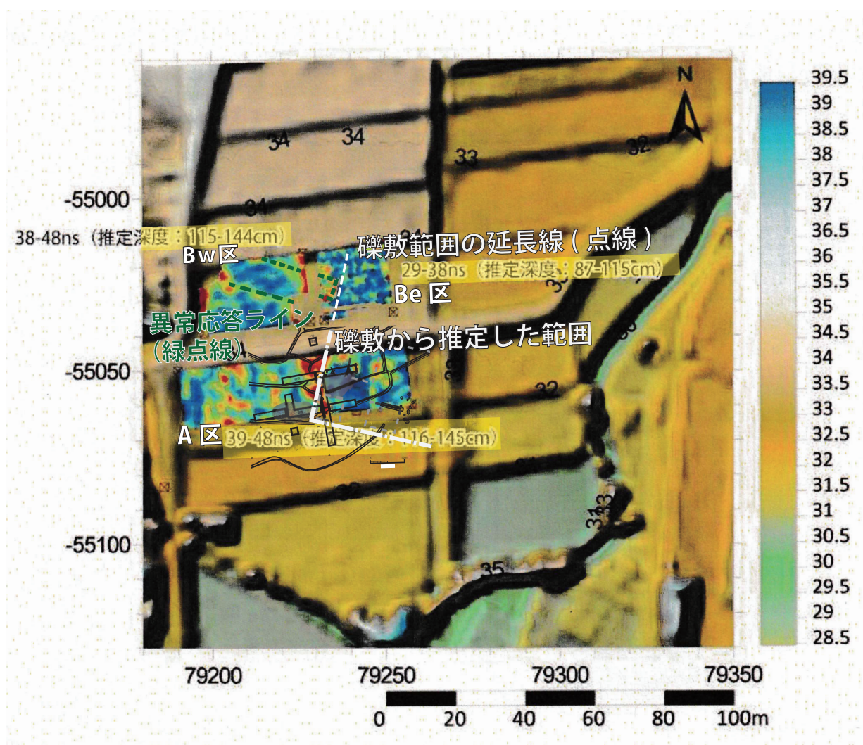
図3 平ノ前廃寺における代表的な地中レーダ探査結果と礫敷想定範囲・異常応答ラインの一部
