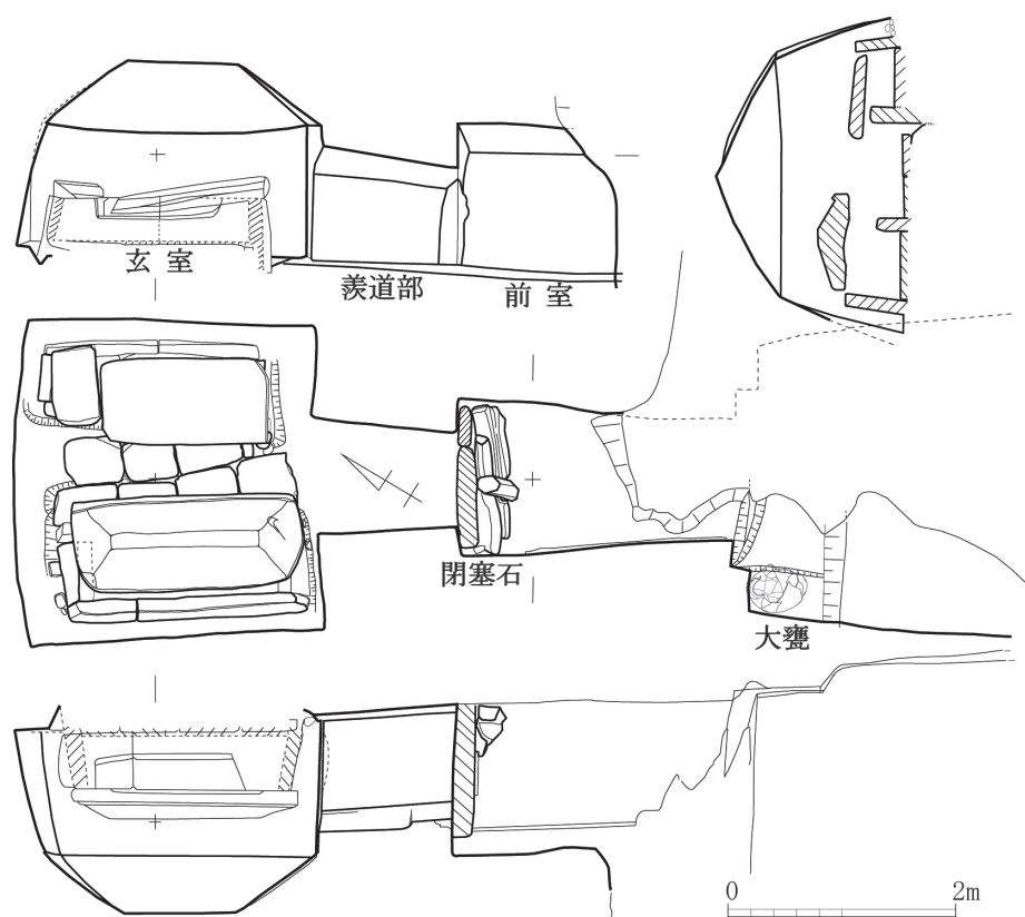
図3 北小原2号横穴墓 実測図
